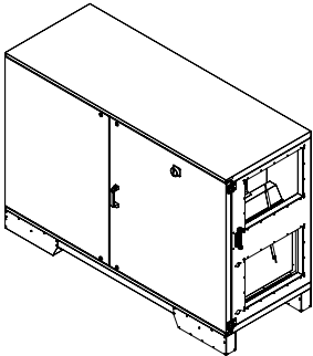
ETA K 2400 H Warmwasserheizregister
