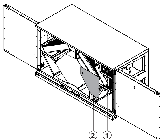
Abb. 12: Anschlussraum (1) Regelplatine (2) Schaltkastendeckel
