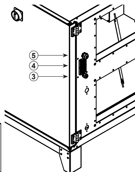
Abb. 13: Kabeldurchführungen (3) Kabeldurchführung Netzanschluss (4) Kabeldurchführung frei (5) Kabeldurchführung Bedienteil
