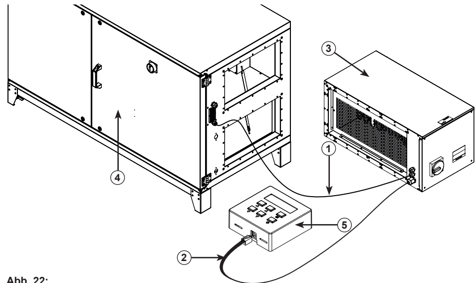
Abb. 22: Anschluss des Bedienteils an das Heizmodul
