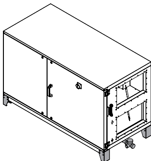
Abb. 10: ETA K 1200 H mit Kugelsiphon
