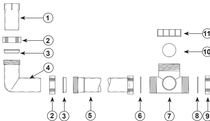
Abb. 11: Systemskizze Kugelsiphon SYS 01
