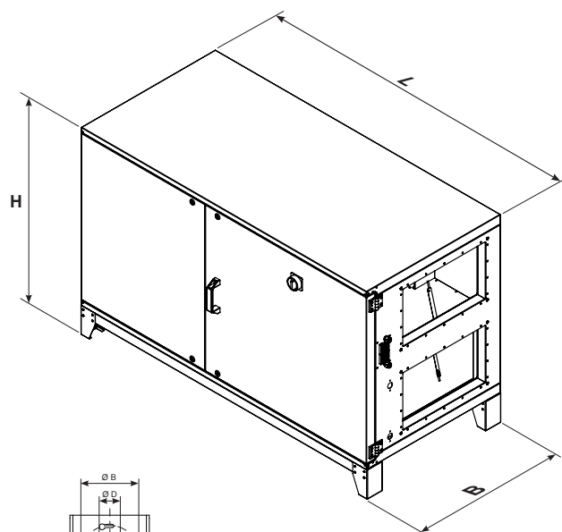
Abb. 27: Abmessungen des Gerätes. ETA K...H
