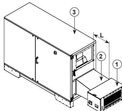
Abb. 21: Anschluss EHM an ETA K 2400 HE
