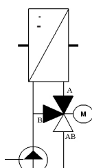
Abb. 6: Umlenk-schaltung
